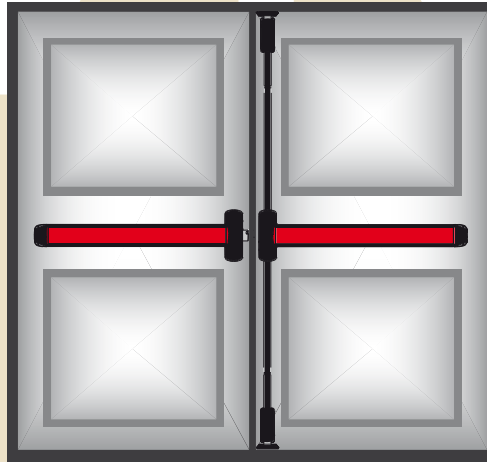
Puertas con contacto mas una falleba
